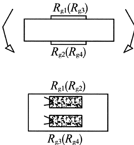
题 32 图 跨中应变片布置方案
